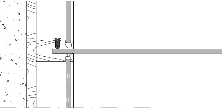
Sezione laterale della mensola in vetro Lateral section of the glass shelf
