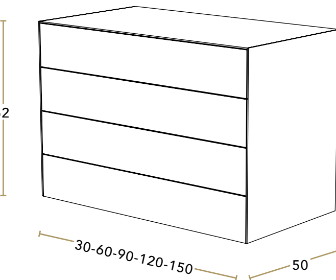
Cassettiera 4 cassetti fissa Fixed 4 drawer-unit
