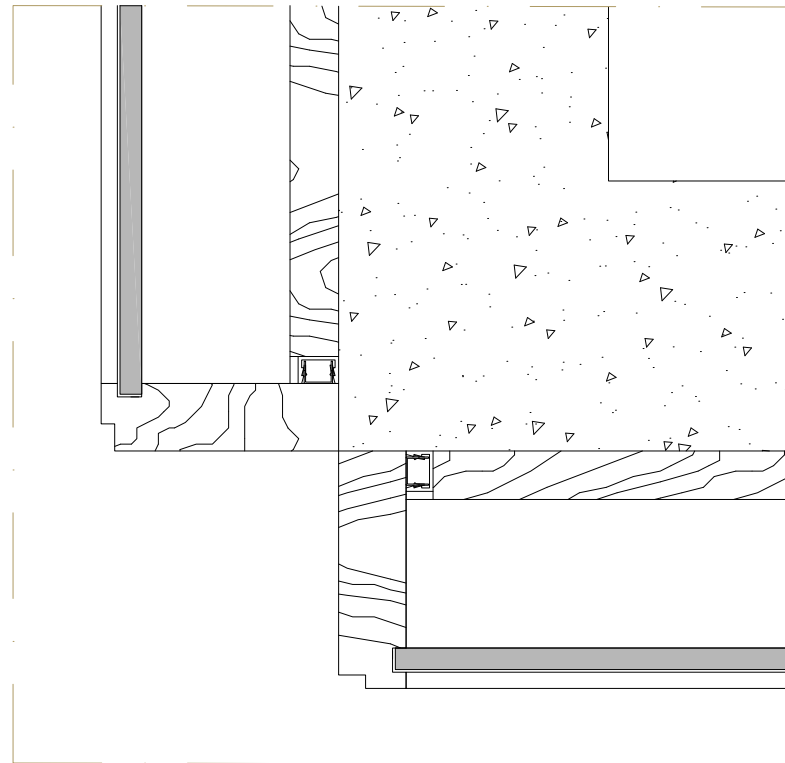
Sezione dell'angolo esterno Section of the external corner
