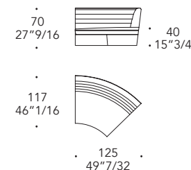
Corner 45°
