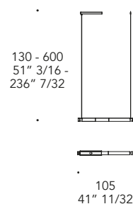
Module 105
