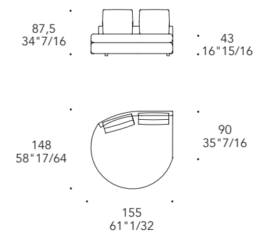
Z - Penisola tonda sx
