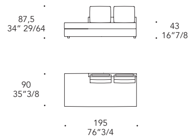
I - Penisola cm. 195 sx
