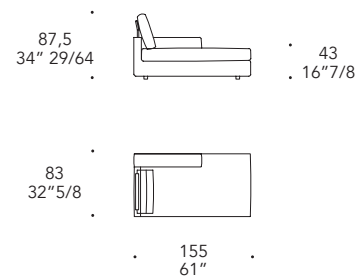
O - Chaise Longue
