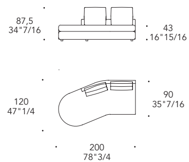
Y - Penisola sagomata sx
